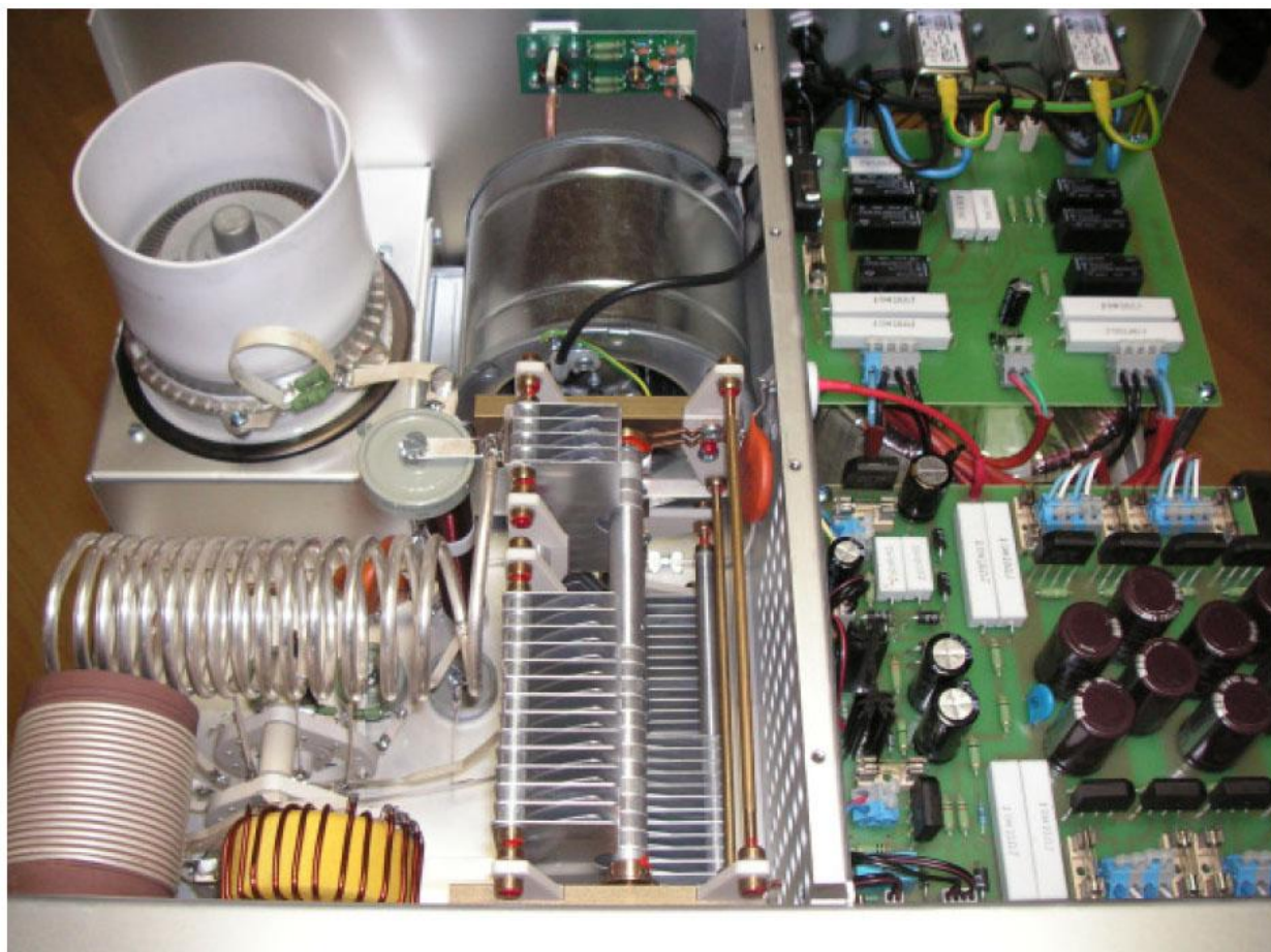
Вид открытого усилителя сверху
